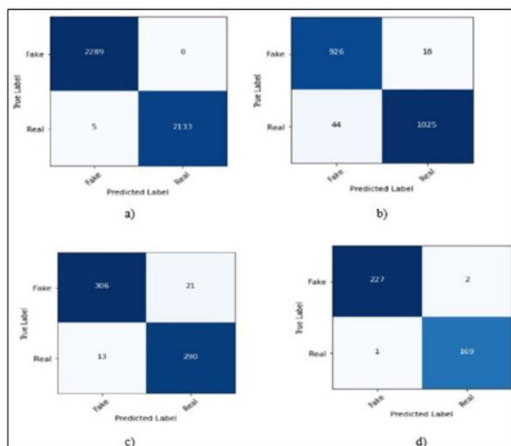
รูปที่ 5 เน้นย้ำประสิทธิภาพของโมเดล ALBERT ในการตรวจจับข่าวปลอม โดยแสดง Confusion Matrices (เมทริกซ์ความสับสน)
